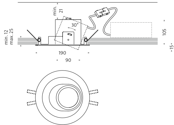
Deckenausschnitt Ceiling cut-out Ø 180 mm
