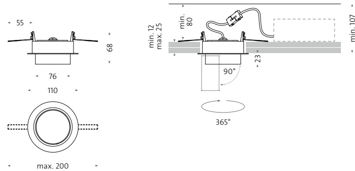
Deckenausschnitt Ceiling cut-out Ø 100 mm
