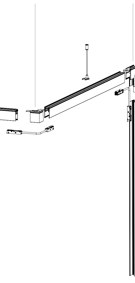
Mechanischer Verbinder 90°, horizontal Mechanical connector 90°, horizontal HW000766 mts-ab-lc-ho
