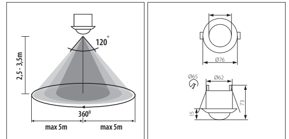
Technische tekening
